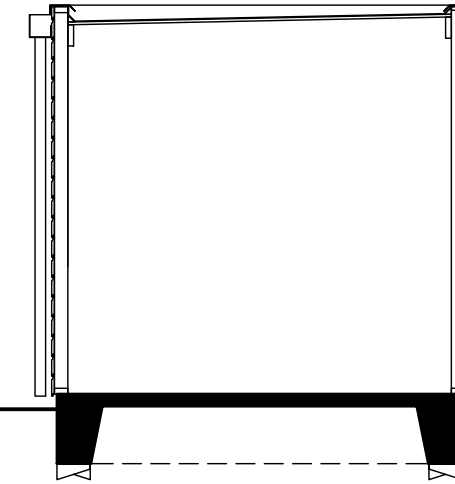
zijgevel
